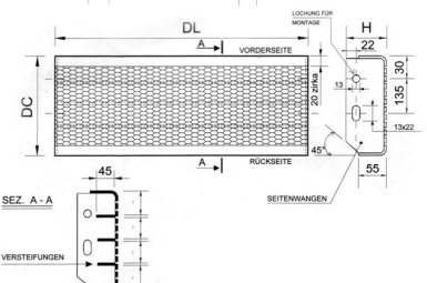
PODEST 43 X 10 DEBELINA 3 mm
