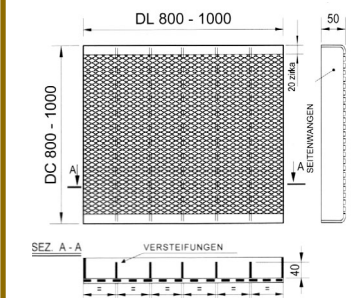
PODEST 43 X 10
