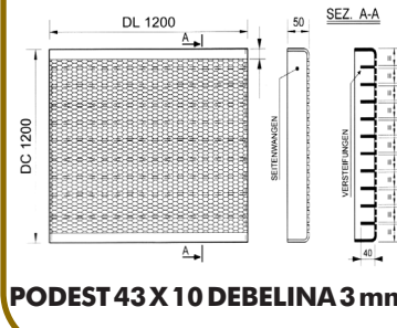
PODEST 43 X 10
