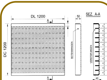
PODEST FELDKIRCH
