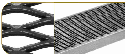
43 x 10 DEBELINA 3 mm
